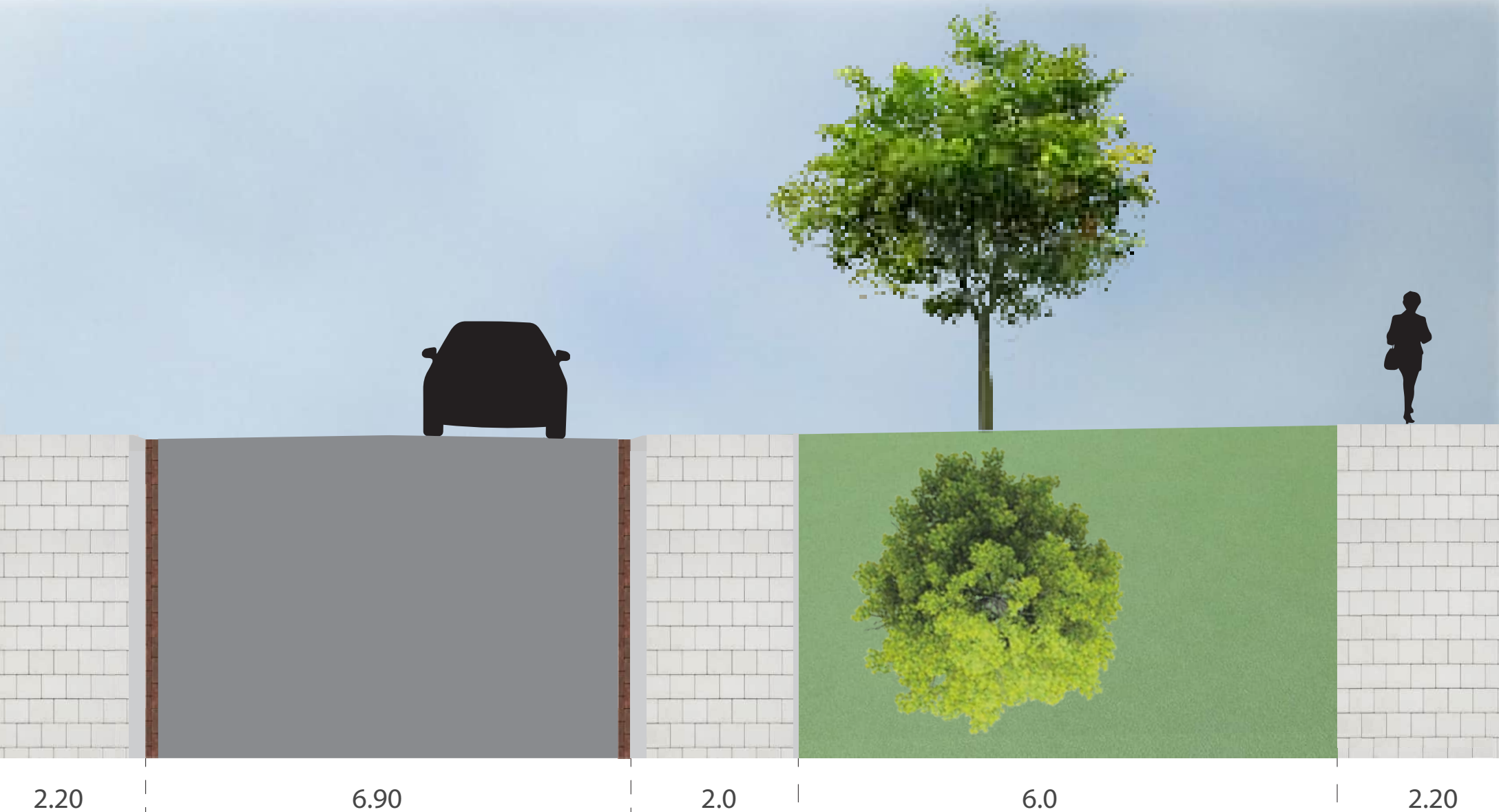
DOORSNEDE B-B'
