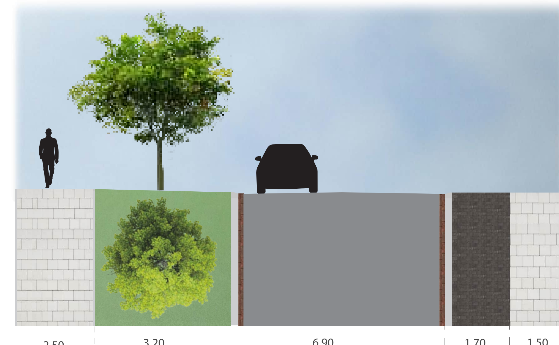
DOORSNEDE A-A'
